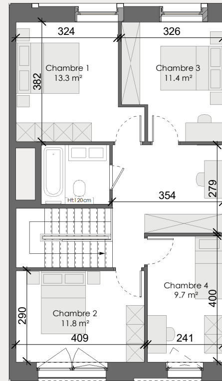
1 er étage (70 m 2 )
