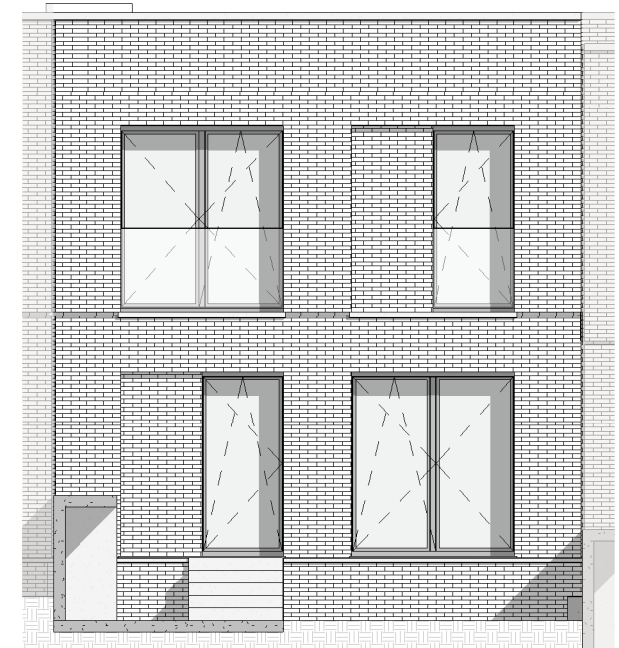
Façade Avant
