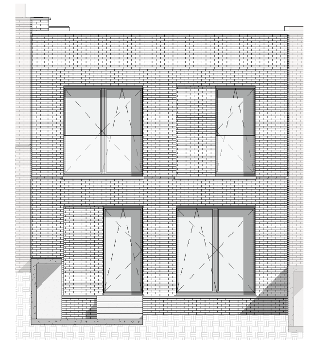
Façade Avant
