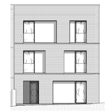
Façade Avant
